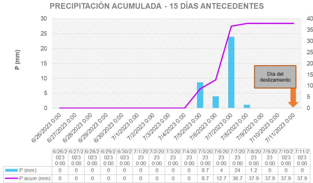
Figura 8. Precipitación antecedente.
