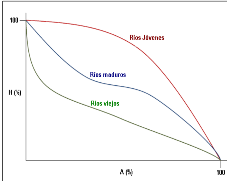
Figura 56 Edad de los ríos de acuerdo a la forma de la curva Hipsométrica, Fuente: (Ibáñez, Ascensio, 2004).
