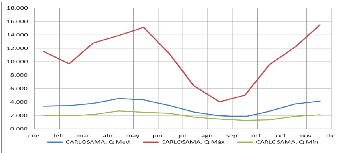
Figura 67 Caudales medios, máximos y mínimos (m³/s) en la estación Carlosama. Fuente: Equipo técnico POMCA
