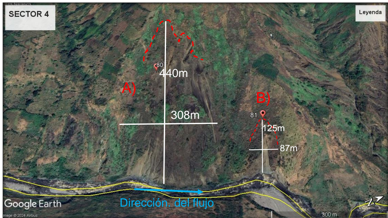
Figura 55 Deslizamientos rotacionales retrogresivos en inmediaciones del municipio de Ancuya vereda Los Naranjos.
