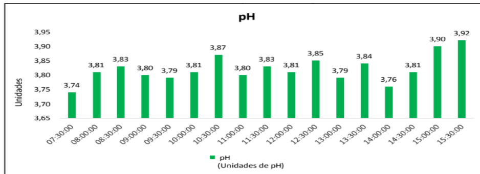
Figura 2: Comportamiento del pH a la salida del STAR
