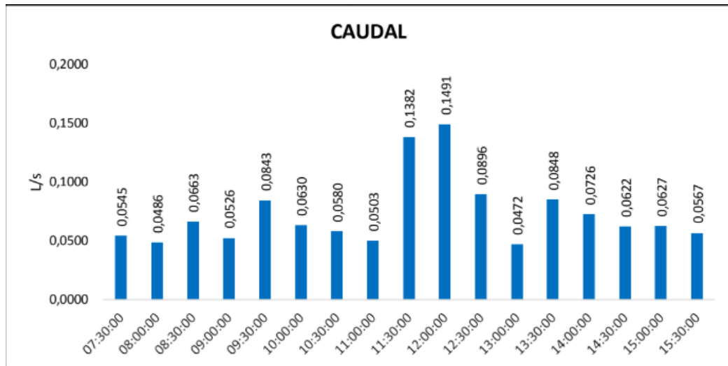
Figura 1: Comportamiento del caudal a la salida del STAR
